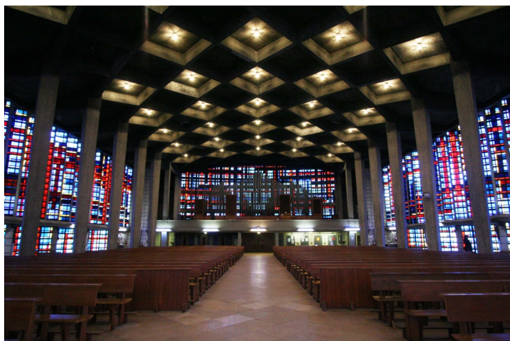
L'église est couverte d'une voûte incurvée en béton constituée de multiples caissons.
